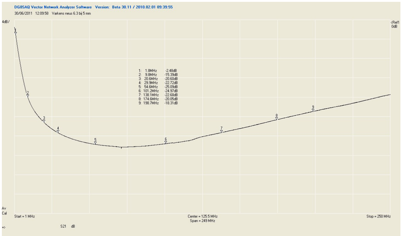
Afbeelding 4: 4 windingen
