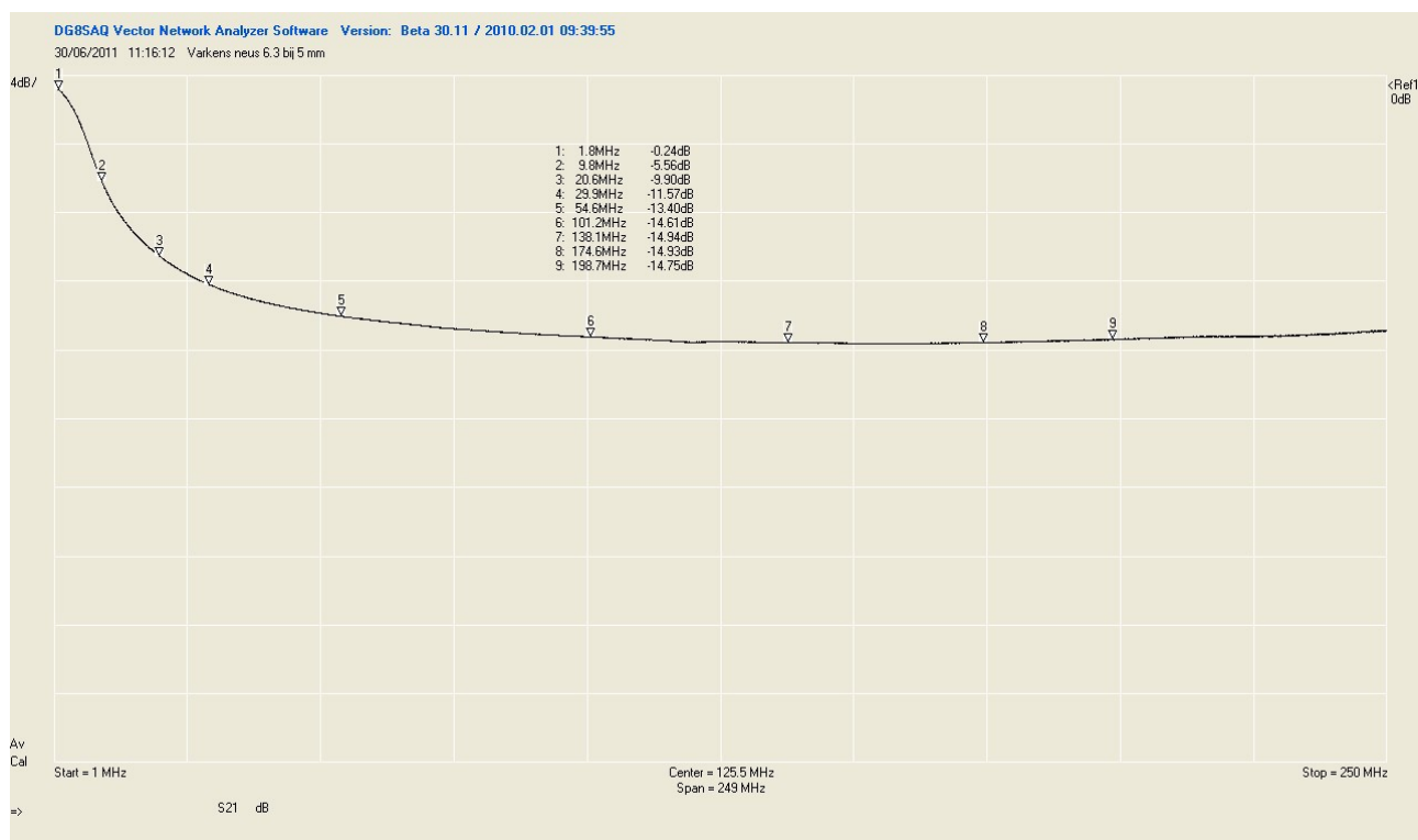
Afbeelding 2: 2 windingen
