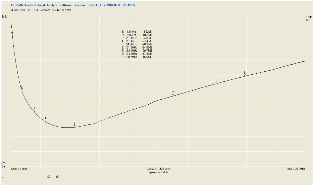
Afbeelding 5: 5 windingen
